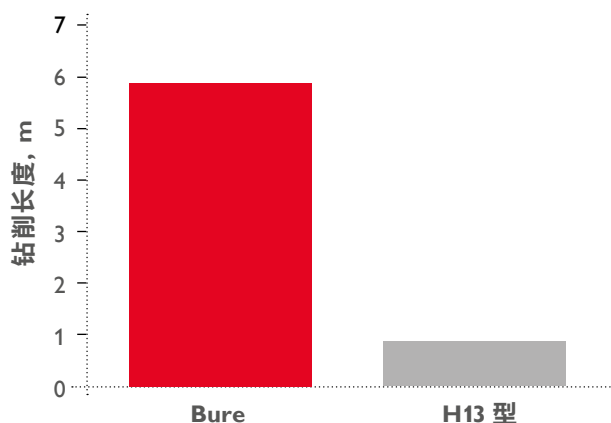
软退火材料中的冷却通道可钻孔长度
